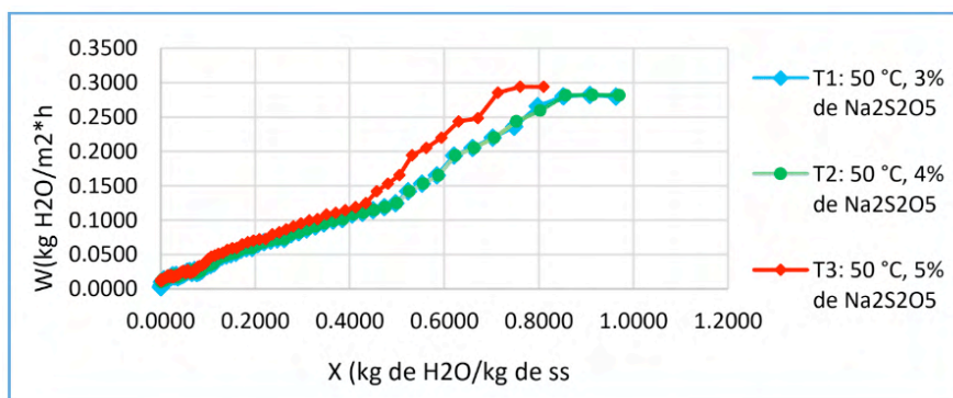
Figura 05: Curva de velocidad de secado a 50 °C. Las curvas describen 2 fases la constante y la decreciente. Gráfico obtenido en el software EXCEL de Microsoft Office (2016)
