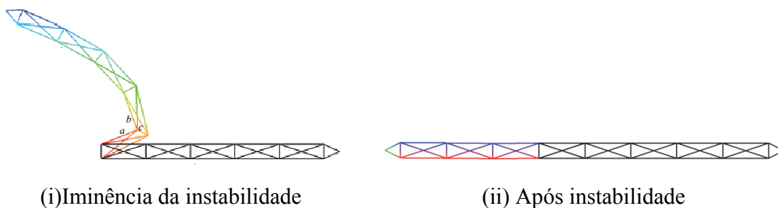
Figura 2.d.6 - Posições deslocadas para modelo de Almansi - Instabilidade
