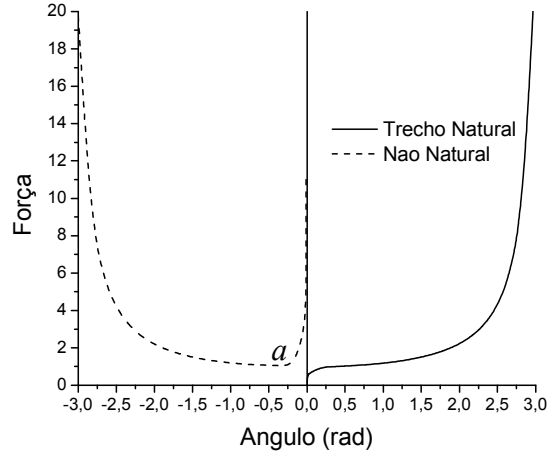
Figura c4 – Força aplicada em função da posição \theta
