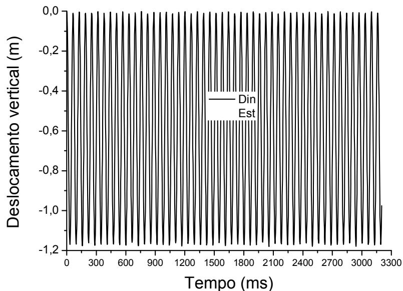
Figura c4 - Deslocamento vertical ao longo do tempo para carga 10x a original
